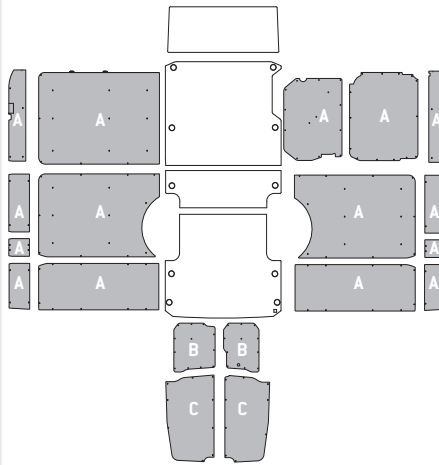
Modello - Modèle L3L H2 - 4100L H2 B
