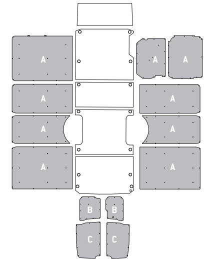
Modello - Modèle L3L H3 - 4100L H3 B
