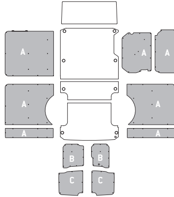
Modello - Modèle L2L H3 - 3520L H3 A
