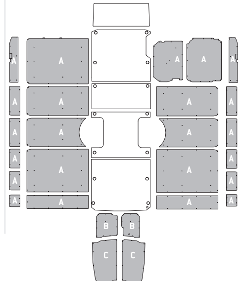
Modello - Modèle L3L H3 - 4100L H3 B
