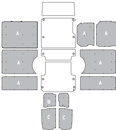
Modello - Modèle L3 H3 - 4100 H3 A
