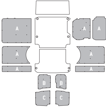
Modello - Modèle L1 H1 - 3000 H1 A
