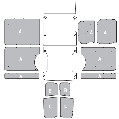
Modello - Modèle L3 H2 - 4100 H2 A
