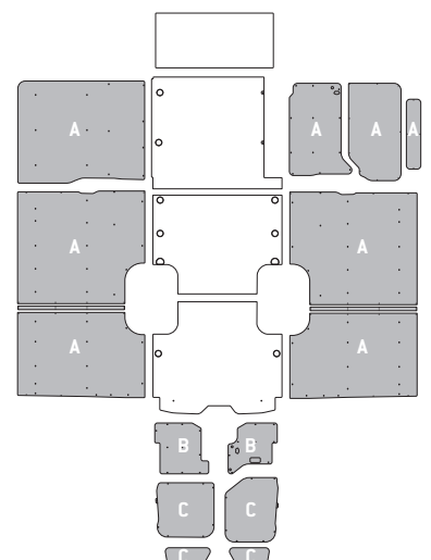
Modello - Modèle L4 H2/H3 C
